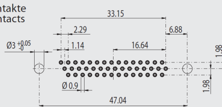
62 Kontakte Contacts
