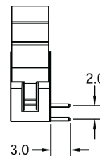
EJECTOR LATCH CAP (AVAILABLE)
