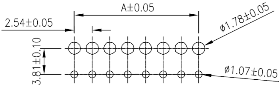
P.C.B LAYOUT
