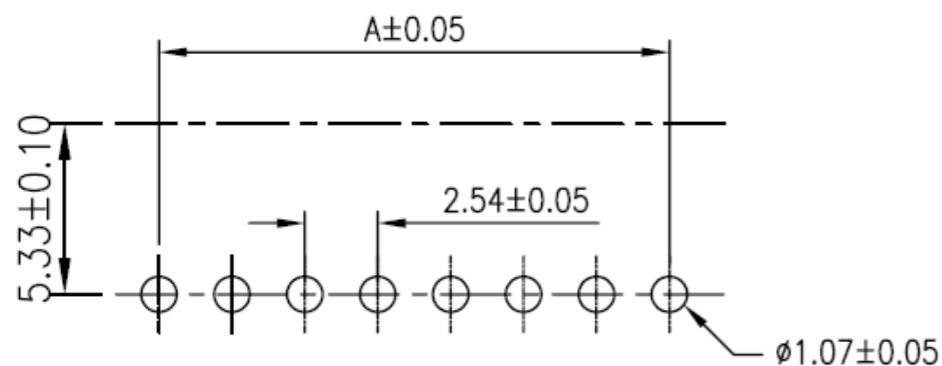
P.C.B LAYOUT
