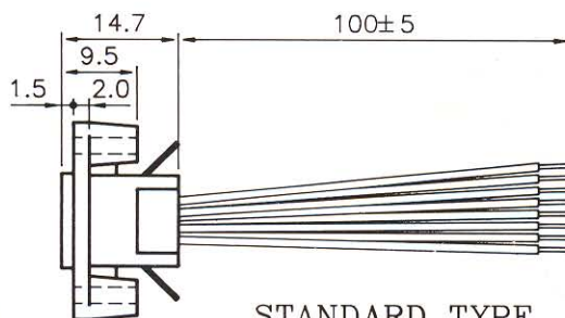
STANDARD TYPE (MDC-163~MDC-168)
