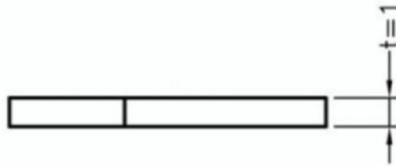
HOLE IN P.C.B \phi 3.0
