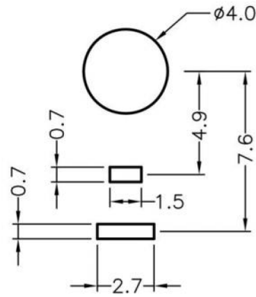
HOLE IN P.C.B
