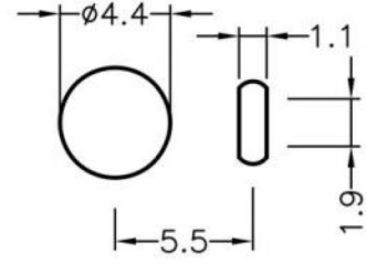
HOLE IN P.C.B
