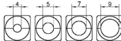
Grommet Sizes MHD45PPK 9-37:
