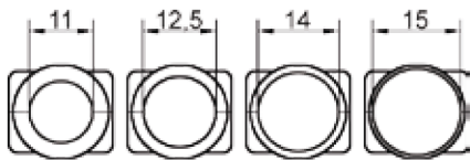
Grommet Sizes / MHD45ZK50
