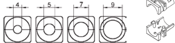
Grommet Sizes / MHD45ZK09-37
